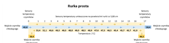
Rys.9. Rozkład temperatur na długości radiatora z rurką prostą
