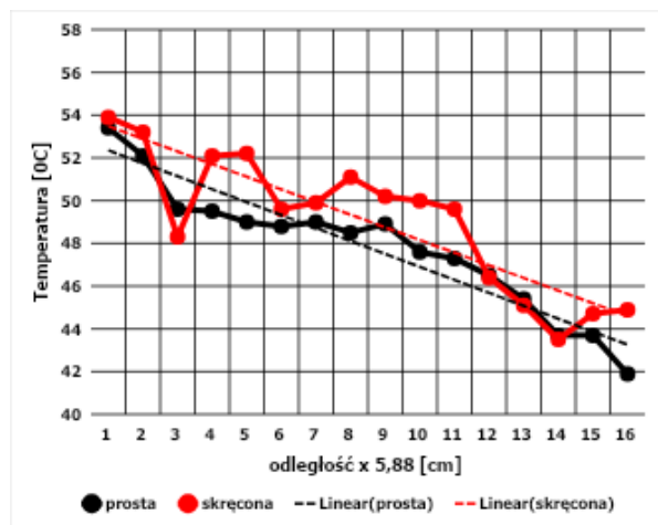
Rys.8. Wyniki pomiarów zmian temperatury na długości radiatora rurowego, dla punktów oddalonych co 5,88cm, dla rurki skręconej (linia czarna) i rurki prostej (linia czerwona), zaznaczono linie trendu przebiegu zmian.
